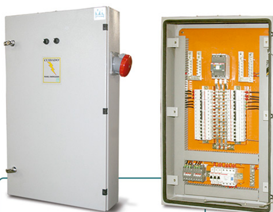
Quadros de Distribuição TTA/PTTA
